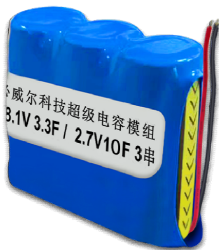
(模组实物图片)
